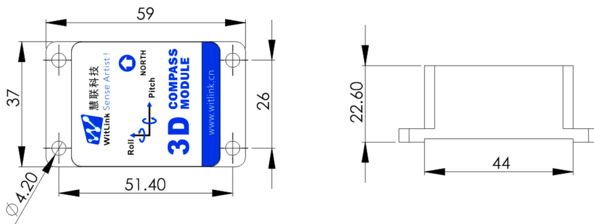
产品尺寸：L59 x W37 x H22.6 mm ( SEC345 )
