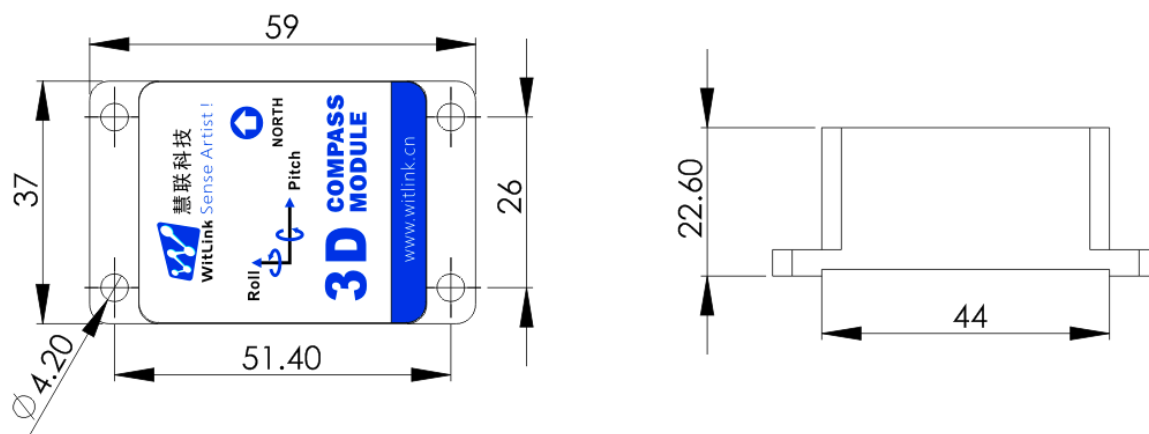
SEC315 产品尺寸：L59 x W37 x H22.6 (mm)
