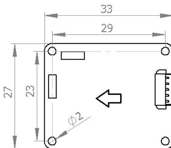
SEC310 产品尺寸：L33 x W27 x H6 (mm)
